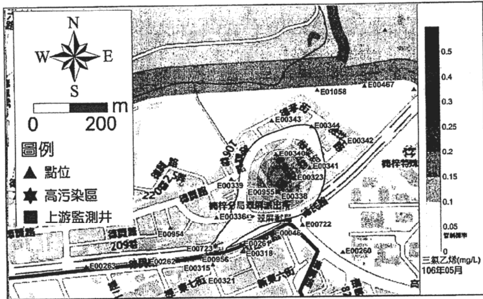
圖 1 桶梓加工出口區東北側區外 TCE 等濃度繪製圖 (水文地質補充調查後)(106年5月)
