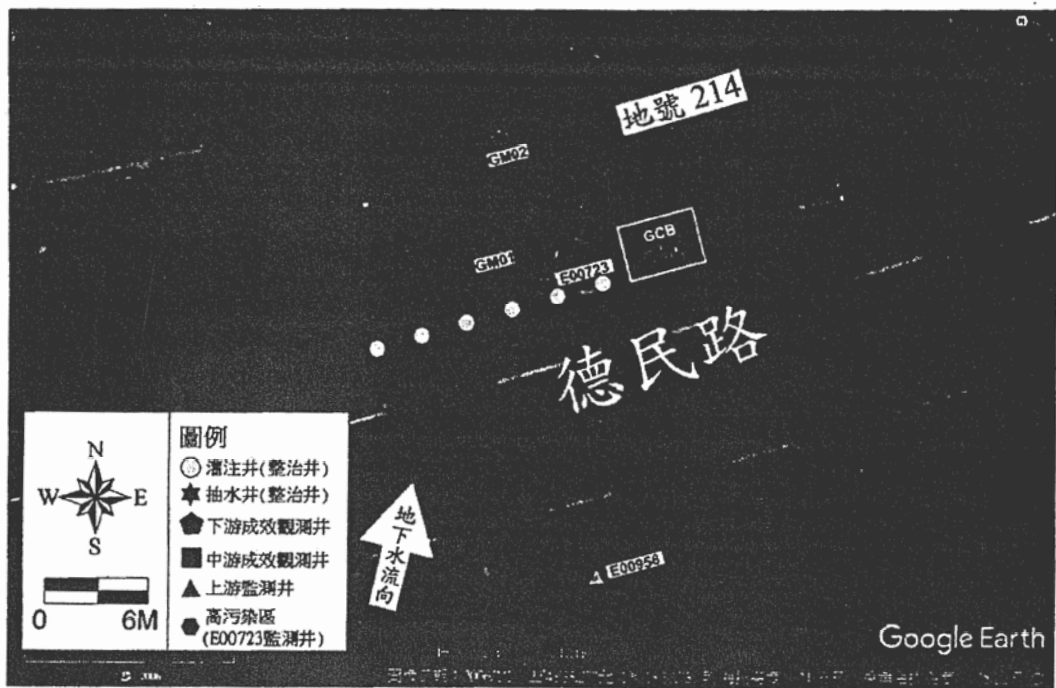
圖 3 高污染區(E00723 監測井)GCB 系統平面配置圖
