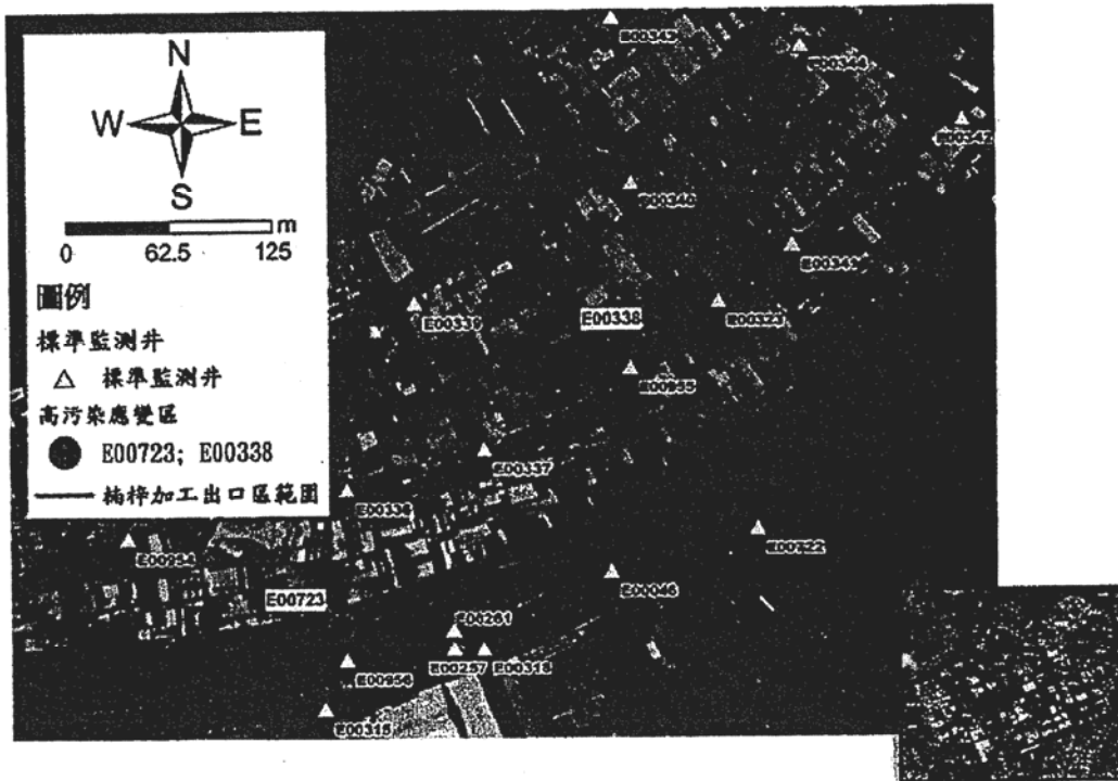
圖 1 桶梓加工出口區東北側區外 TCE 等濃度繪製圖 (水文地質補充調查後)(106年5月)
